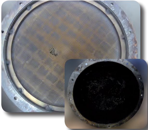
Ein beschädigter und ein verschmutzter Filter.
